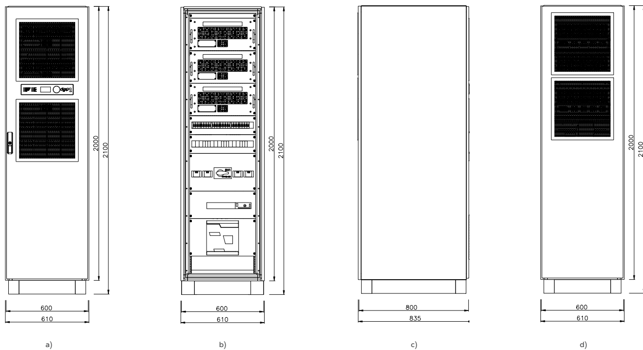
Rys. 91. Widoki z wymiarami szafy UPS MODULA:
