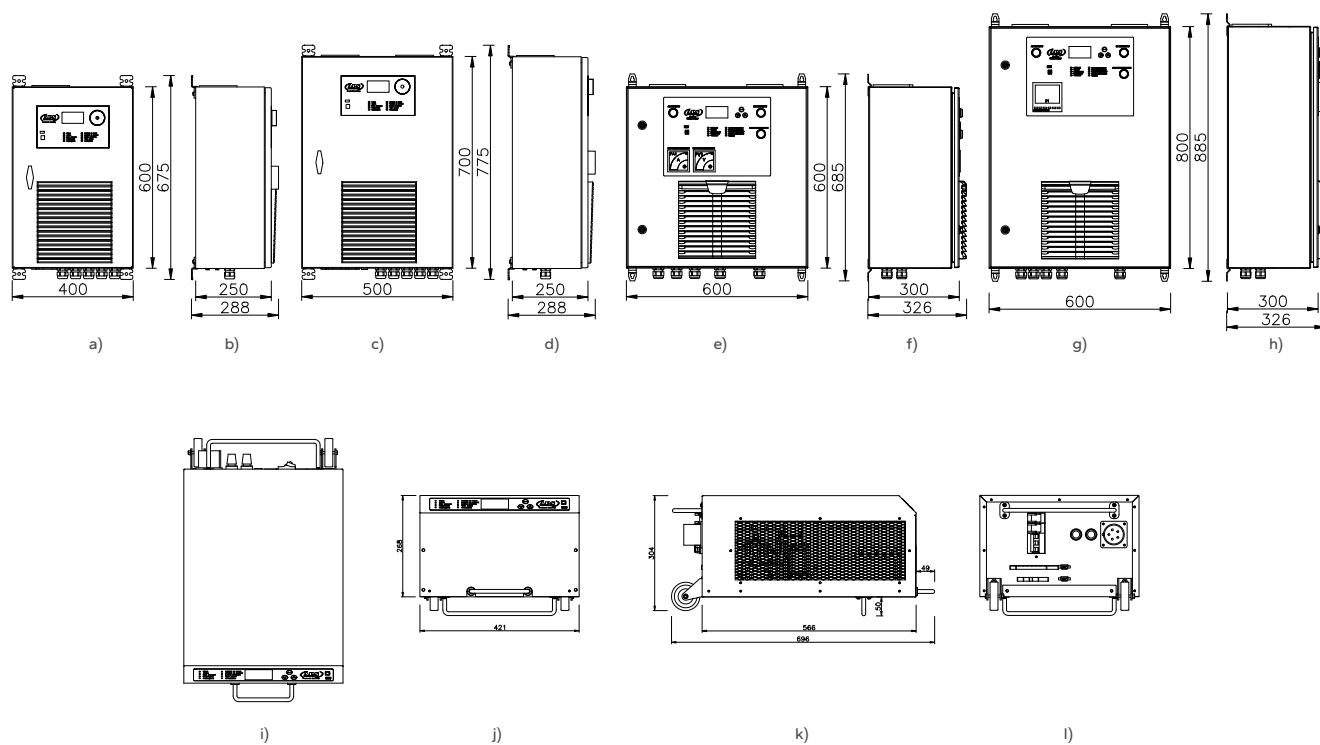
Rys. 19. Widoki z wymiarami kompaktu prostownika typu PBI (obudowa wisząca i przenośna):
