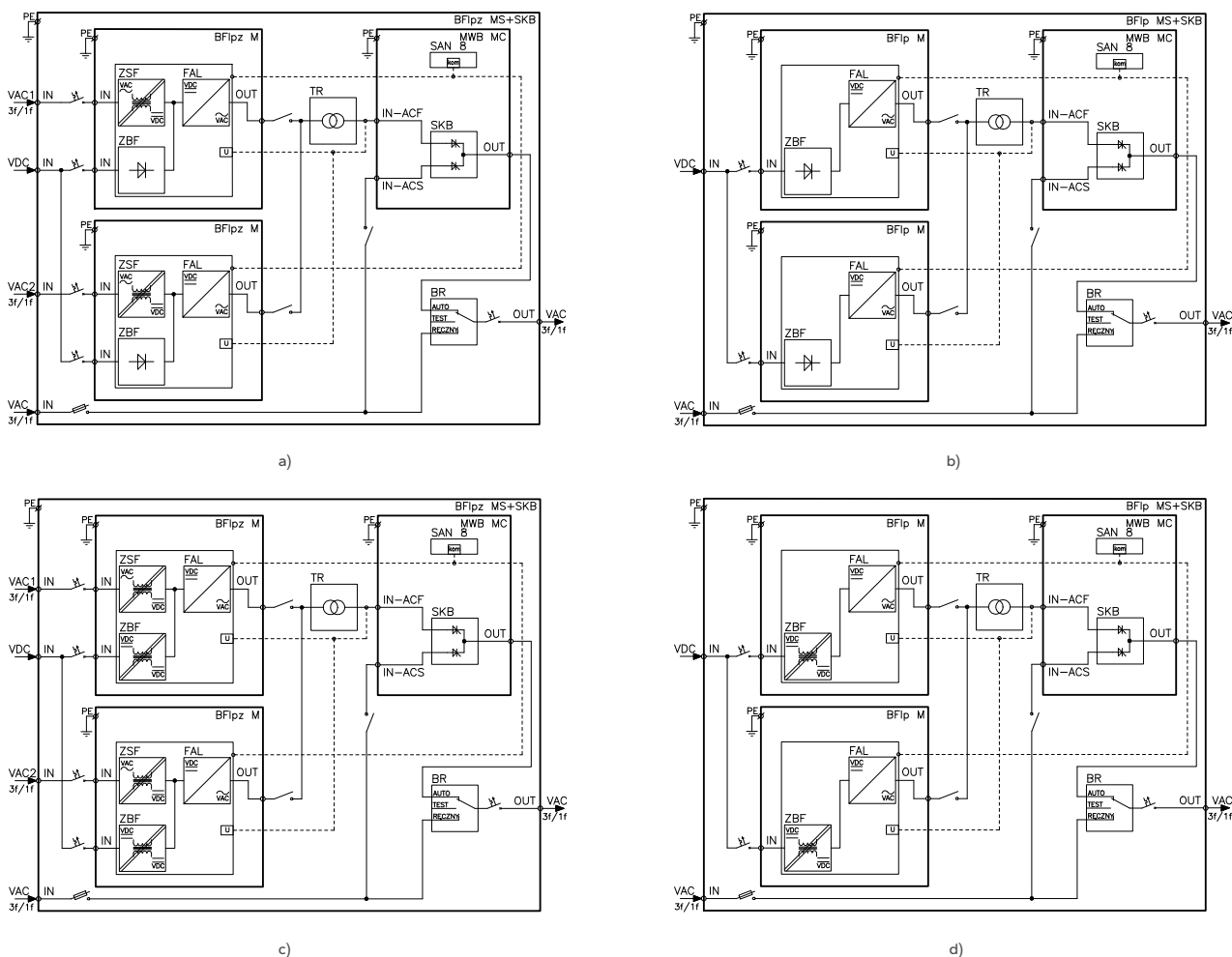
Rys. 64. Schemat blokowy szafy falownika składającej się z modułów falownika do pracy równoległej typu BF1pz / BF1p o max mocy modułu do 10 kVA wraz z bypassem typu SKB oraz wspólnym transformatorze (rozwiązanie 1-fazowe lub 3-fazowe). Możliwe konfiguracje:
