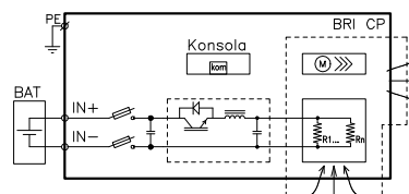
Rys. 42. Schemat blokowy kompaktu opornicy rozładowczej typu BRI.
