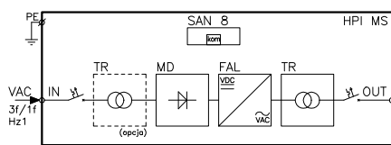
Rys. 96. Schemat blokowy szafy przetwornicy częstotliwości swobodnej zabudowy:
