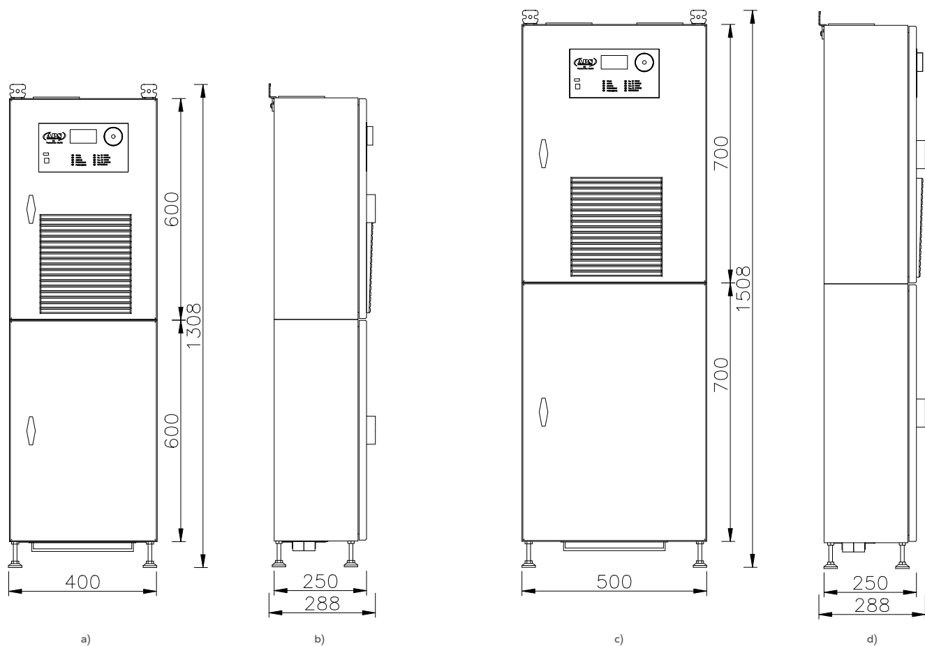
Rys. 40. Widoki z wymiarami kompaktu przetwornicy typu EPI (obudowa stojąca):
