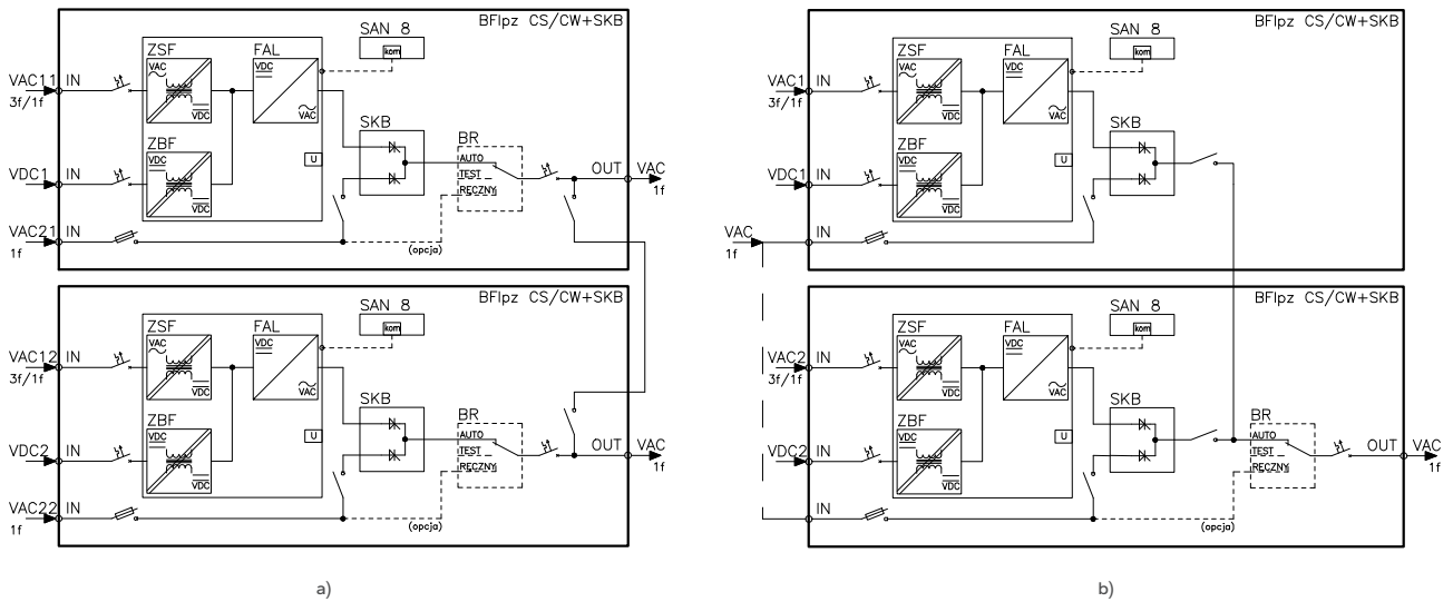
Rys. 74. Schemat blokowy kompaktów falownika do pracy równoległej z zasilaczem sieciowym typu BFIp oraz bypassem typu SKB. Możliwe konfiguracje: a) dwa niezależne przełączniki bypasu remontowego, zabudowana konsola; b) wspólny przełącznik bypasu remontowego, zabudowana konsola.
