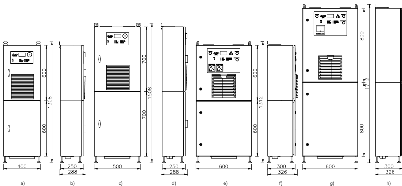
Rys. 18. Widoki z wymiarami kompaktu prostownika typu PBI (obudowa stojąca):
