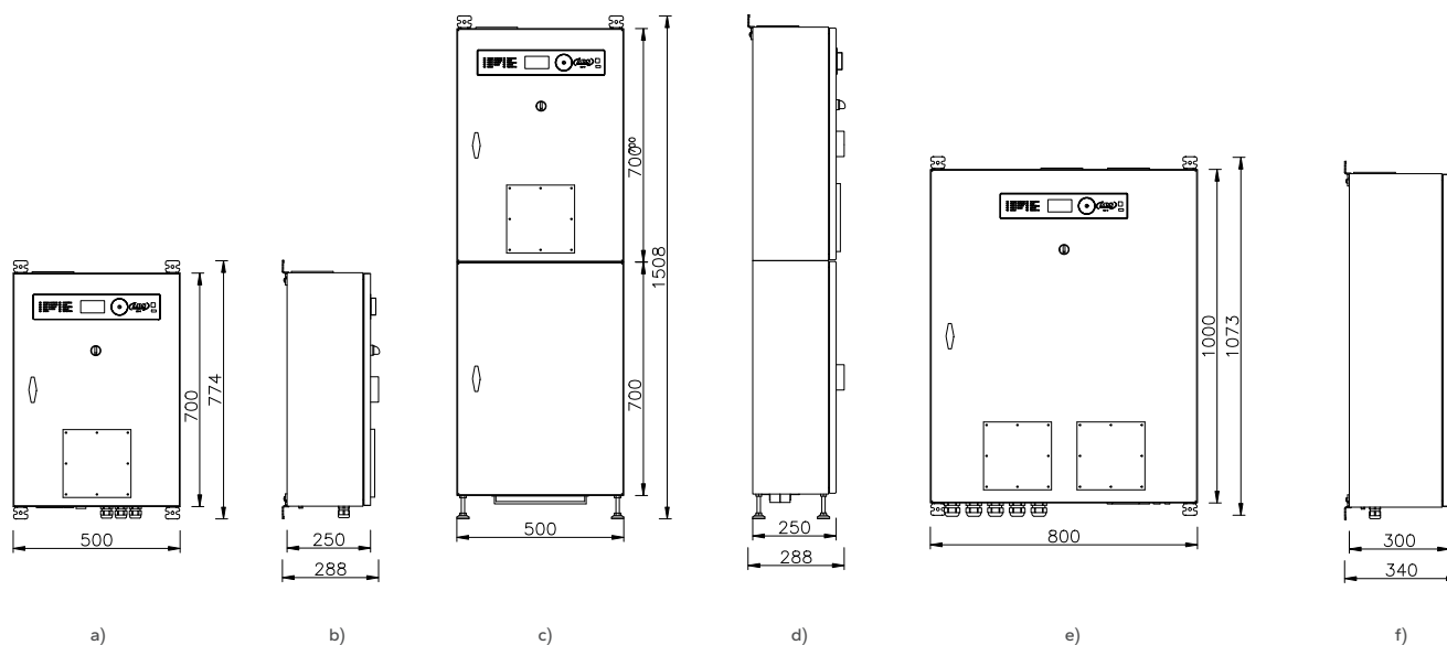
Rys. 73. Widoki z wymiarami kompaktu falownika typu BFIz / BFI:
