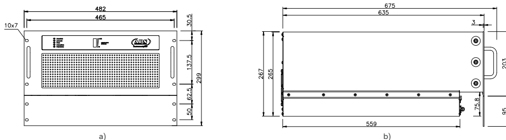
Rys. 103. Widoki z wymiarami modułu falownika napędowego typu FATz / FAT MC: a) widok od przodu w obudowie M5; b) widok z lewej strony w obudowie M5.
