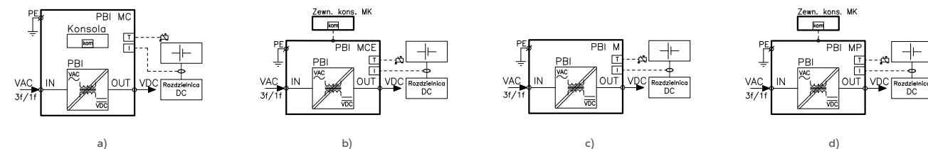
Rys. 7. Schemat blokowy modułu prostownika typu PBI do pracy autonomicznej:
