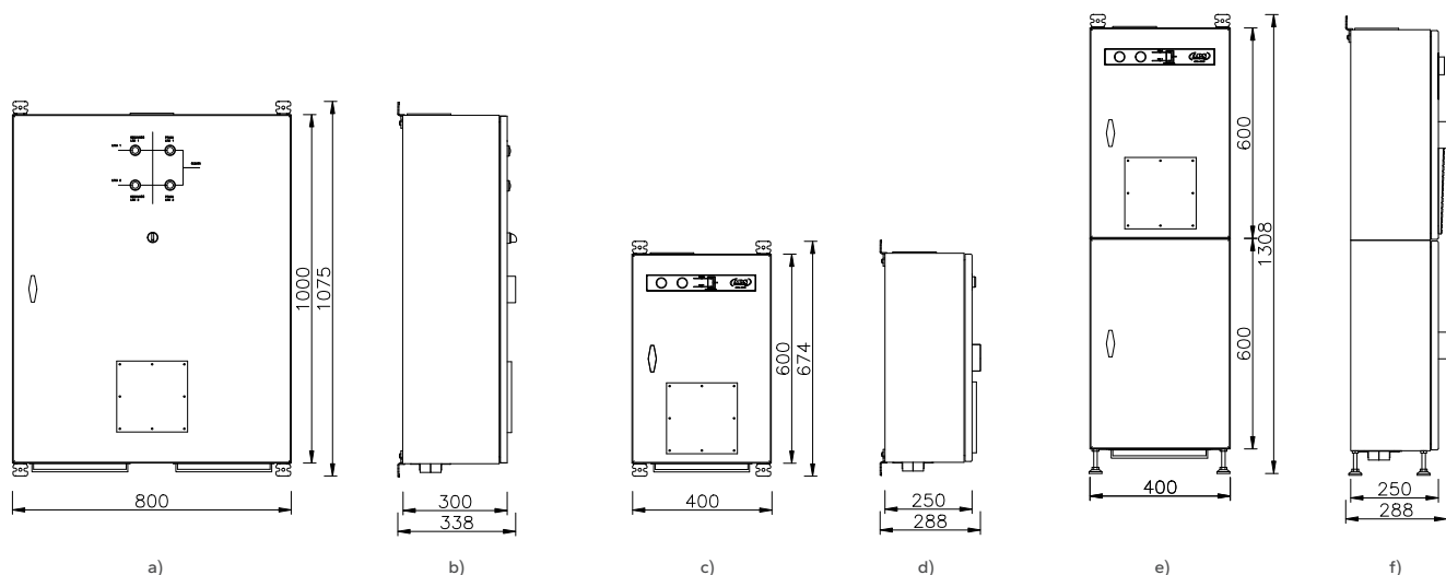
Rys. 86. Widoki z wymiarami kompaktu łącznika statycznego typu SKB:
