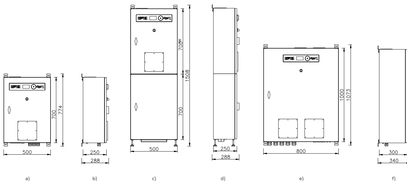
Rys. 76. Widoki z wymiarami kompaktu falownika typu BFlpz / BFIP:
