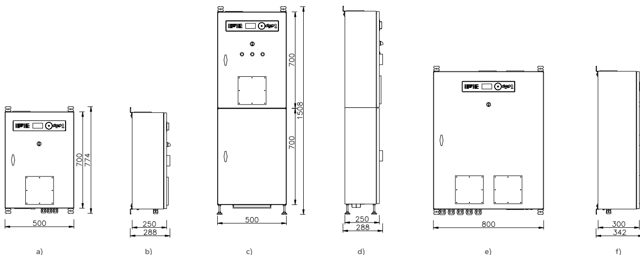
Rys. 99. Widoki z wymiarami kompaktu przetwornicy częstotliwości typu HPI: a) kompakt CW6 – widok od przodu; b) kompakt CW6 – widok z lewej strony; c) kompakt CS6 – widok od przodu; d) kompakt CS6 – widok z lewej strony; e) kompakt CW1 – widok od przodu; f) kompakt CW1 – widok z lewej strony.
