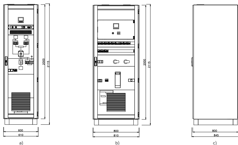
Rys. 84. Widoki z wymiarami szafy łącznika statycznego typu SKB:
