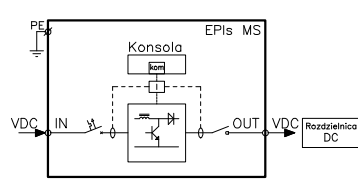
Rys. 34. Schemat blokowy szafy przetwornicy typu EPIs do pracy autonomicznej: a) zabudowa modułowa; b) zabudowa swobodna.
