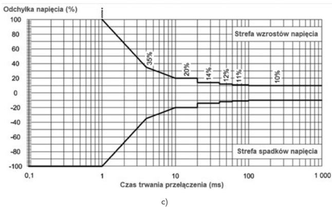
Rys. 79. Charakterystyka błędów napięcia linii: a) typ APS4; b) wg normy EN62040 – 3 Class 1; c) EN62040 – 3 Class 2; d) EN62040 – 3 Class 3.
