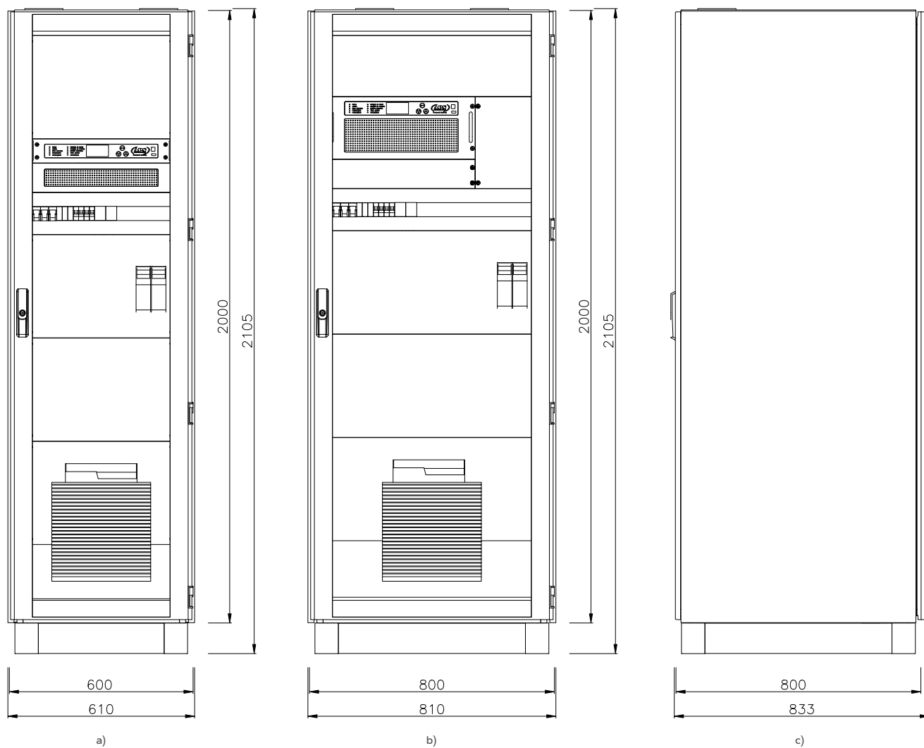
Rys. 15. Widoki z wymiarami szafy prostownika typu PBI:
