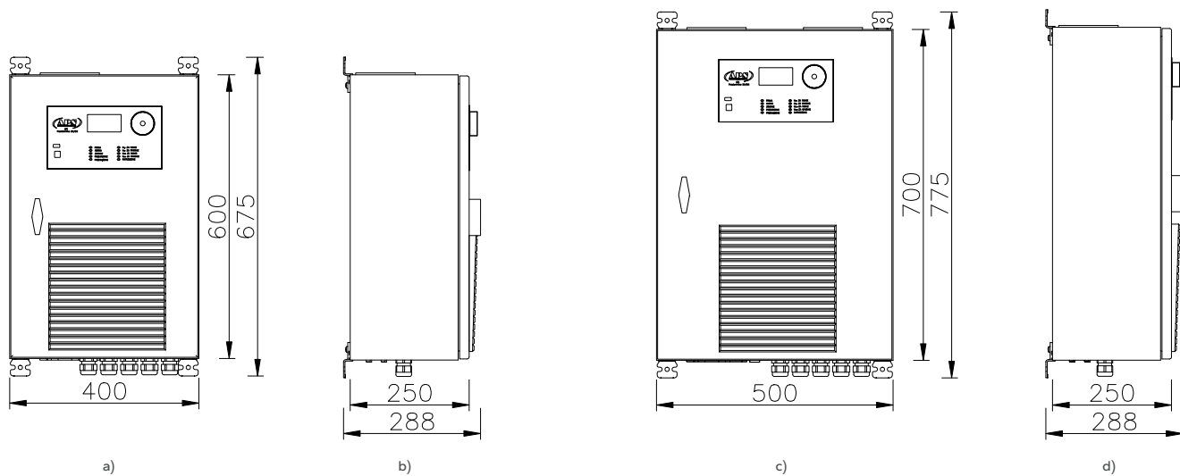
Rys. 41. Widoki z wymiarami kompaktu przetwornicy typu EPI (obudowa wisząca):
