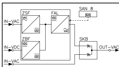
Rys. 44. Ogólny schemat blokowy układu falownikowego z zasilaczem sieciowym typu BFIz oraz bypasssem typu SKB
