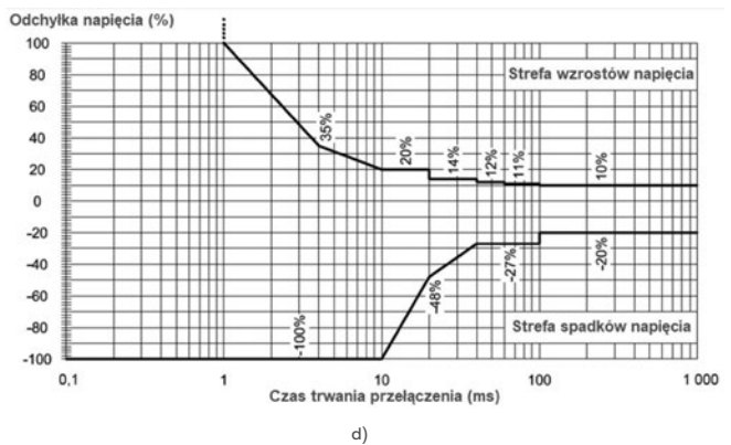
Rys. 79. Charakterystyka błędów napięcia linii: a) typ APS4; b) wg normy EN62040 – 3 Class 1; c) EN62040 – 3 Class 2; d) EN62040 – 3 Class 3.
