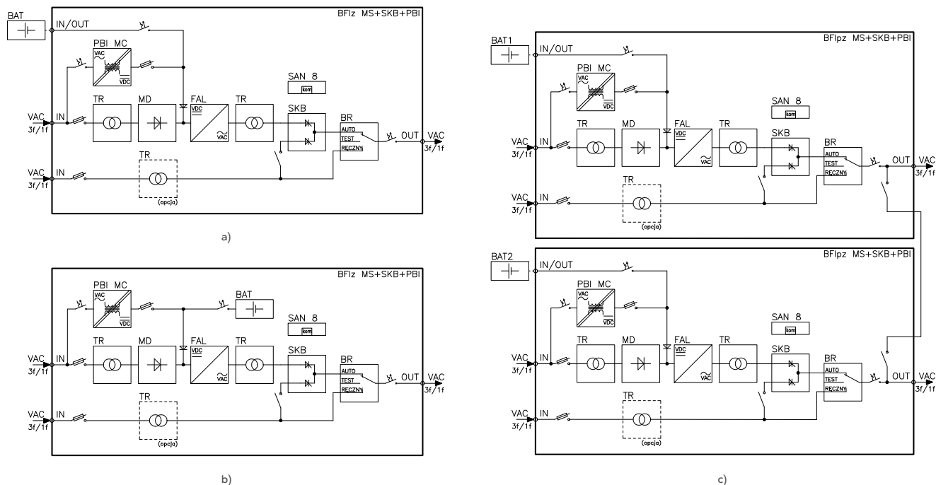
Rys. 87. Schemat blokowy szafy systemu UPS:
