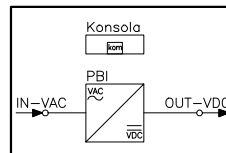
Rys. 1. Ogólny schemat blokowy układu prostownikowego
