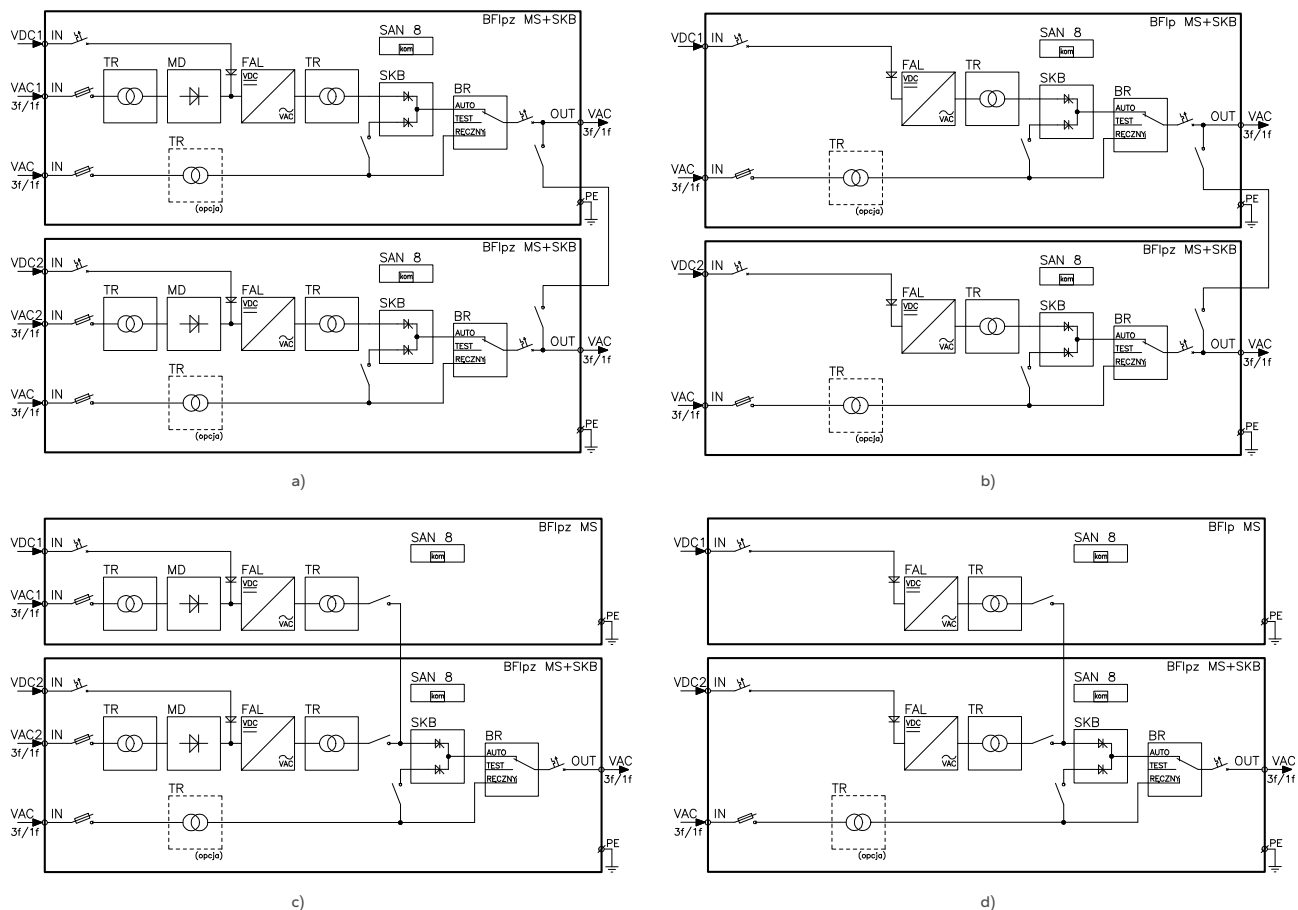
Rys. 67. Schemat blokowy szaf falowników w swobodnej zabudowie do pracy równoległej typu BFlpz / BFlp wraz bypassem typu SKB. Możliwe konfiguracje:
