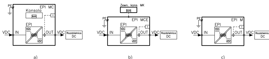
Rys. 27. Schemat blokowy modułu przetwornicy z izolacją galwaniczną typu EPI do pracy autonomicznej:
