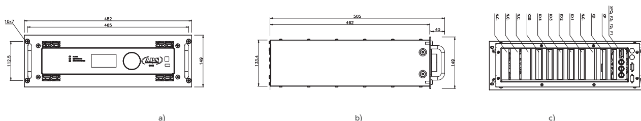
Rys. 108. Widoki z wymiarami modułu systemu automatycznego nadzoru typu SAN 3M:
