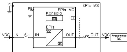
Rys. 34. Schemat blokowy szafy przetwornicy typu EPIs do pracy autonomicznej: a) zabudowa modułowa; b) zabudowa swobodna.
