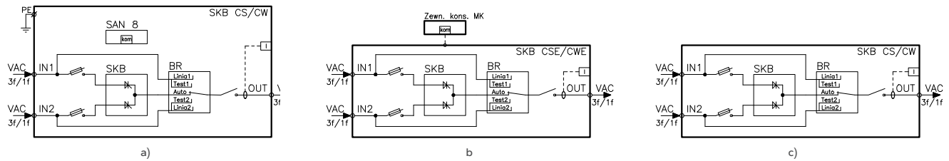
Rys. 85. Schemat blokowy kompaktu łącznika statycznego typu SKB: a) wraz z zabudowaną konsolą; b) wraz z zewnętrzną konsolą MK; c) bez konsoli.
