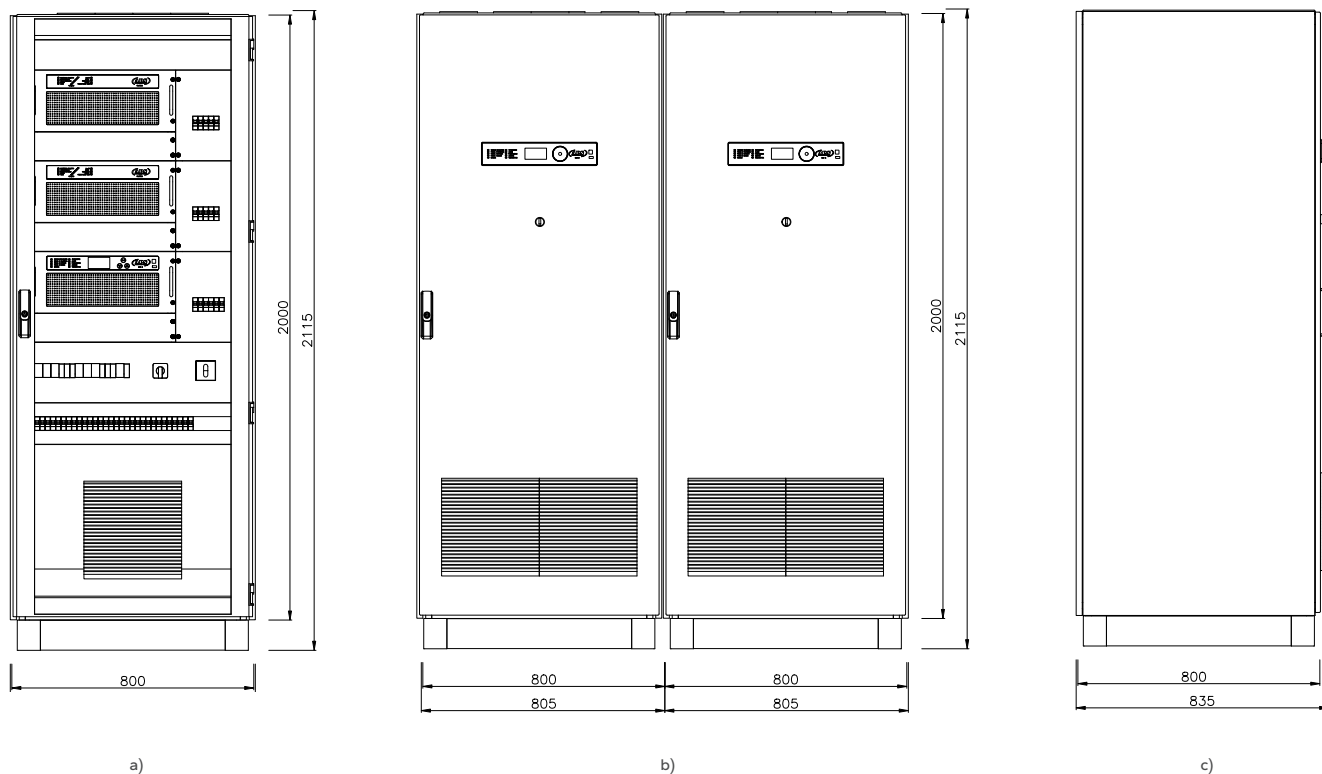
Rys. 69. Widoki z wymiarami szafy falownika typu BFIpz / BFIpz:
