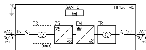
Rys. 96. Schemat blokowy szafy przetwornicy częstotliwości swobodnej zabudowy:
