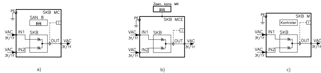
Rys. 80. Schemat blokowy modułu łącznika statycznego typu SKB:
