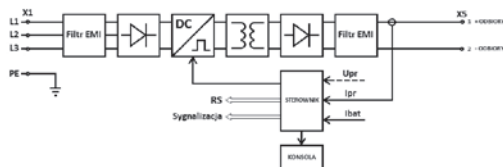
Rys. 2. Schemat ideowy prostownika typu PBI
