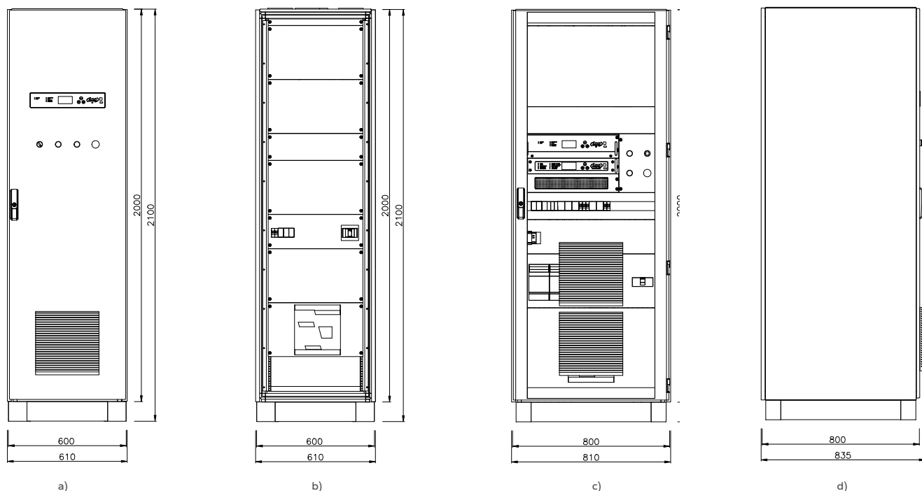
Rys. 105. Widoki z wymiarami szafy systemu zasilania silników asynchronicznych typu FATz / FAT:
