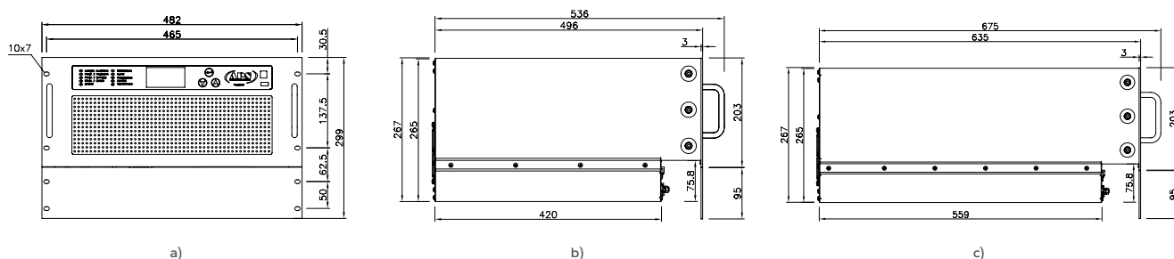
Rys. 48. Widoki z wymiarami modułu falownika typu BFIz / BFI MC (opcjonalnie):
