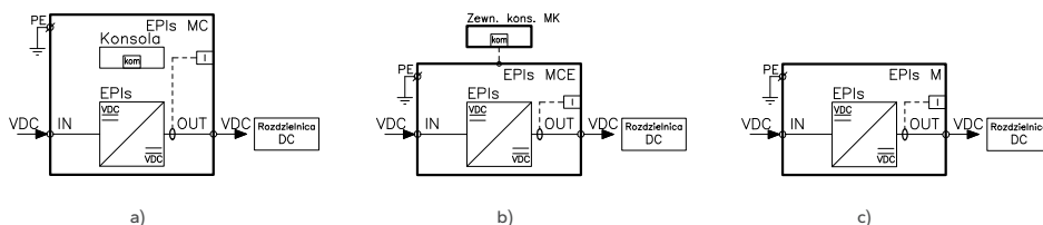
Rys. 28. Schemat blokowy modułu przetwornicy bez izolacji typu EPIs do pracy autonomicznej:
