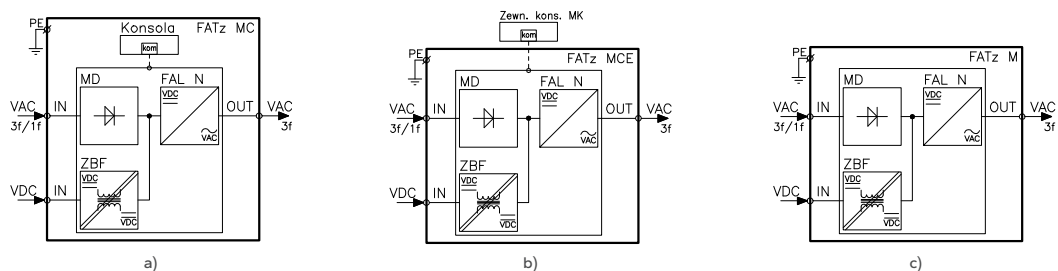
Rys. 101. Schemat blokowy modułu falownika napędowego z zasilaczem sieciowym typu FAT: a) wraz z zabudowaną konsolą; b) wraz z zewnętrzną konsolą MK; c) bez konsoli.
