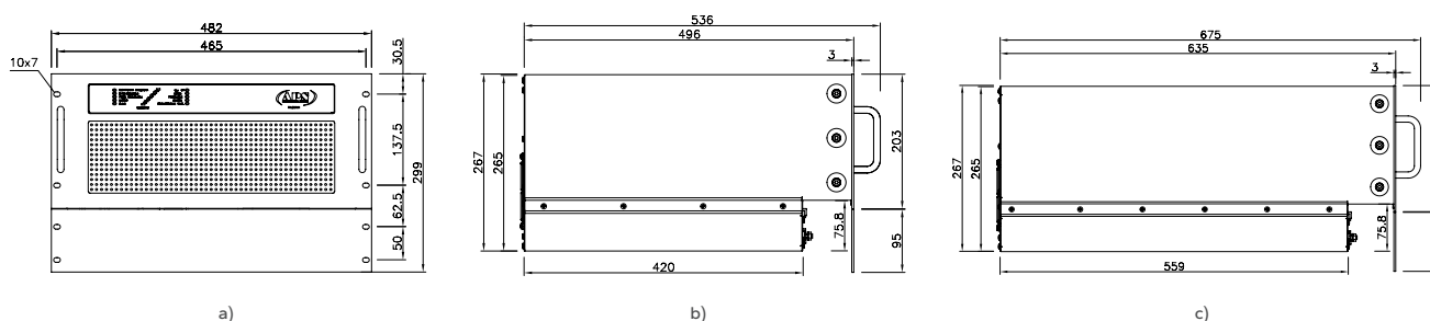
Rys. 57. Widoki z wymiarami modułu falownika typu BFIpz / BFIp M:
