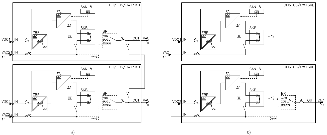
Rys. 75. Schemat blokowy kompaktów falownika do pracy równoległej typu BFIp z bypassem typu SKB. Możliwe konfiguracje: a) dwa niezależne przełączniki bypasu remontowego, zabudowaną konsolą; b) wspólny przełącznik bypasu remontowego, zabudowaną konsolą.
