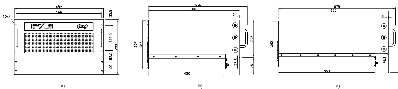
Rys. 54. Widoki z wymiarami modułu falownika typu BFIz / BFI M:
