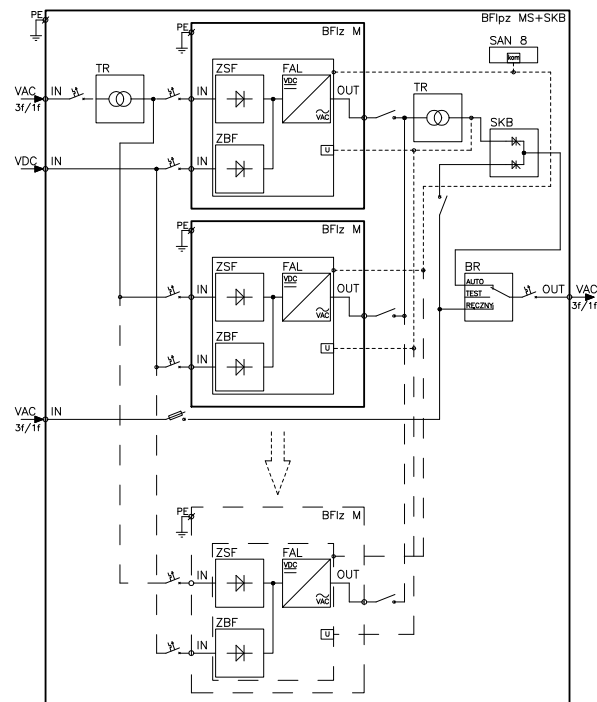
Rys. 66. Schemat blokowy szafy falownika składającej się z modułów falownika do pracy równoległej typu BF1pz o max mocy modułu do 15 kVA wraz z bypassem typu SKB. Układ „n” modułowych falowników ze wspólnym bypassem (rozwiązanie 1-fazowe lub 3-fazowe).
