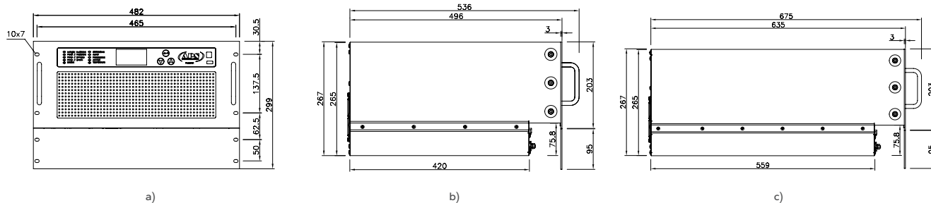
Rys. 58. Widoki z wymiarami modułu falownika typu BFIz / BFI MC HC
