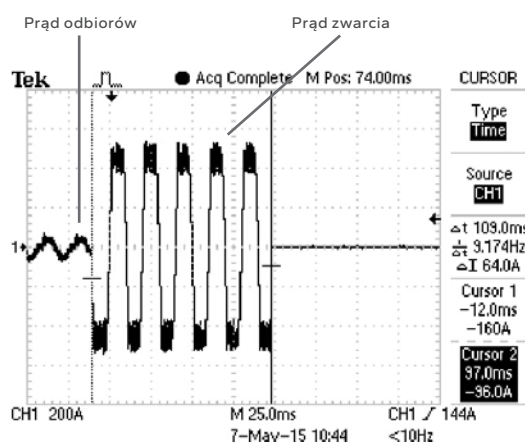
Oscylogram zaprogramowanego prądu i czasu zwarcia falownika
