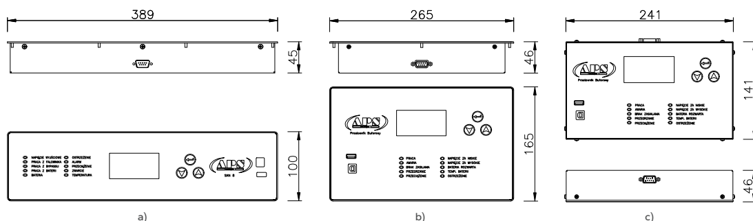
Rys. 106. Widoki z wymiarami konsol przenośnych typu MK: a) konsola K1; b) konsola K2; c) konsola K3.
