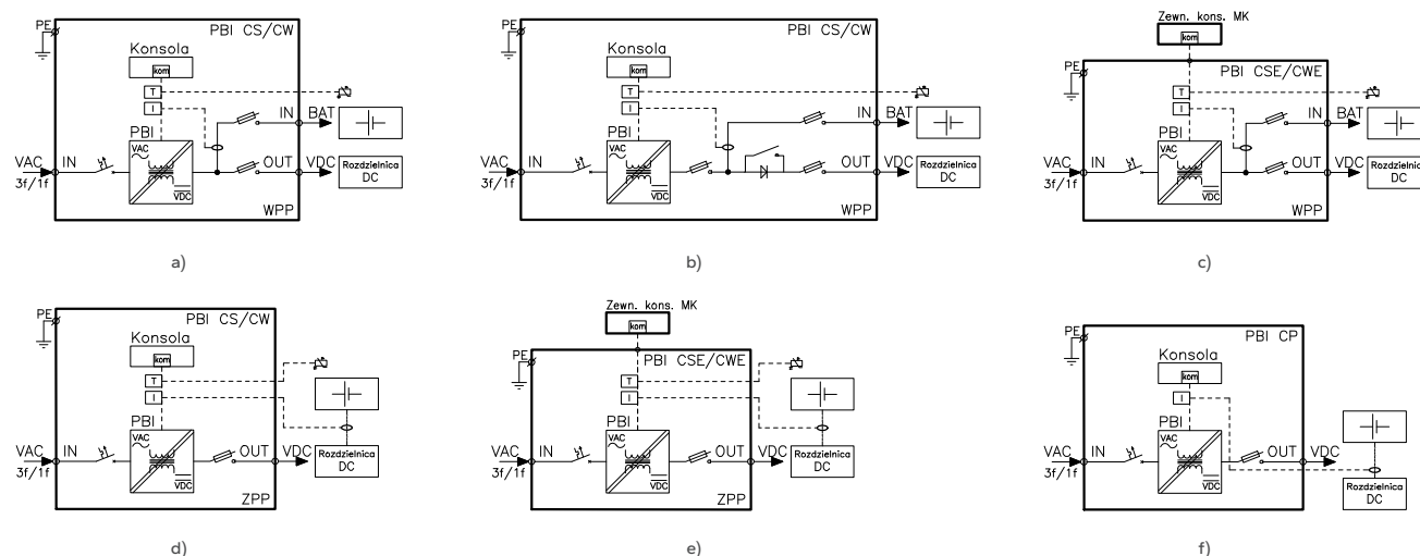
Rys. 16. Schemat blokowy kompaktu prostownika typu PBI do pracy autonomicznej: a) układ z WPP; b) układ z WPP oraz przeciwoogniwem; c) układ z WPP oraz z zewnętrzną konsolą MK; d) układ z ZPP; e) układ z ZPP oraz z zewnętrzną konsolą MK; f) układ kompaktu przenośnego.
