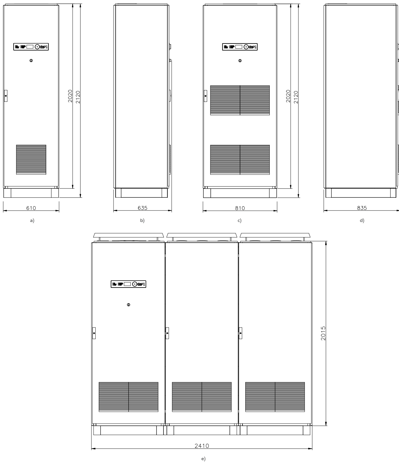
Rys. 21. Widoki z wymiarami szafy prostownika tyrystorowego typu PBI T:
