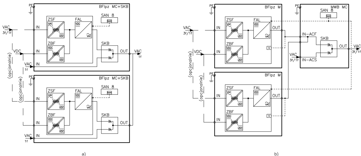
Rys. 49. Schemat blokowy modułów falownika do pracy równoległej z zasilaczem sieciowym typu BFIpz. Możliwe konfiguracje: a) dwa niezależne bypassy typu SKB, zabudowana konsola w module falownika; b) wspólny bypass typu SKB, zabudowana konsola w module MWB.
