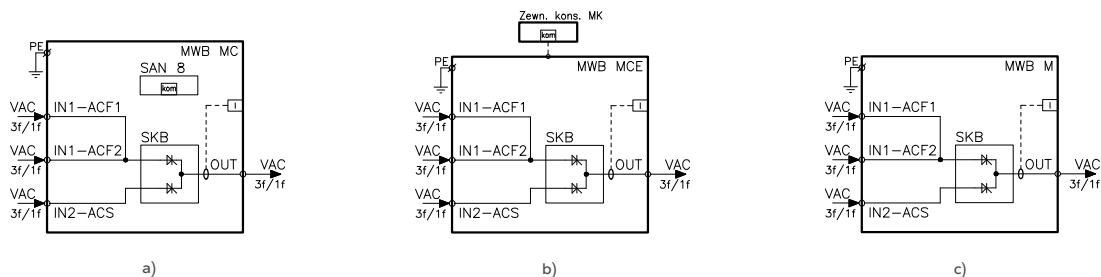
Rys. 81. Schemat blokowy modułu łącznika statycznego typu MWB:
